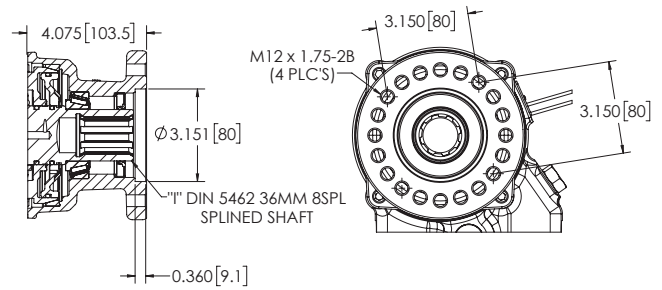
“II” OUTPUT - DIN 5462
